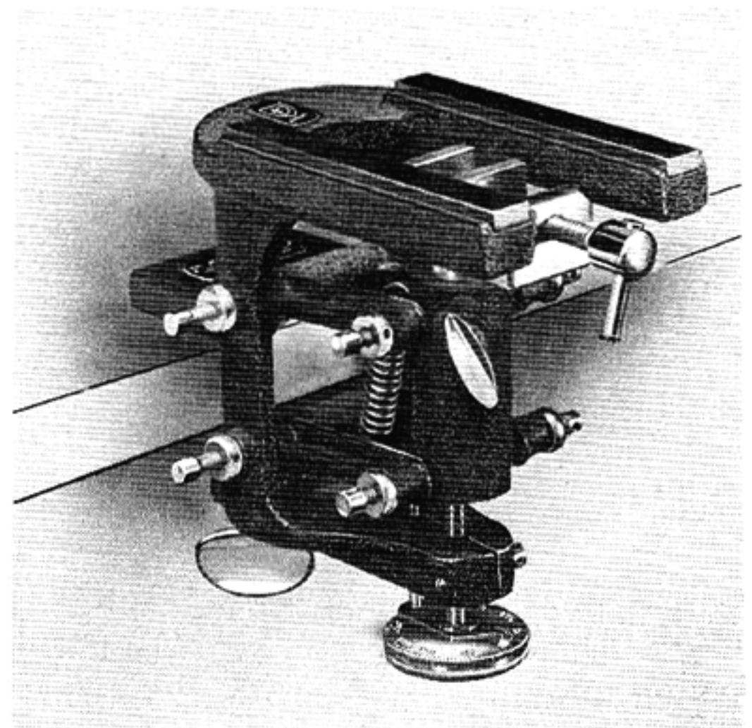
Fig. 16. AO Table Microtome.
