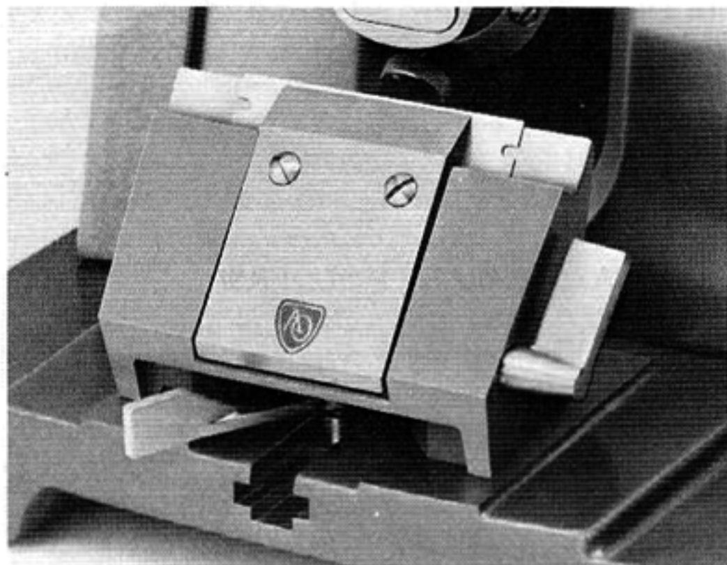
Fig. 24. Disposable Blade Holder
