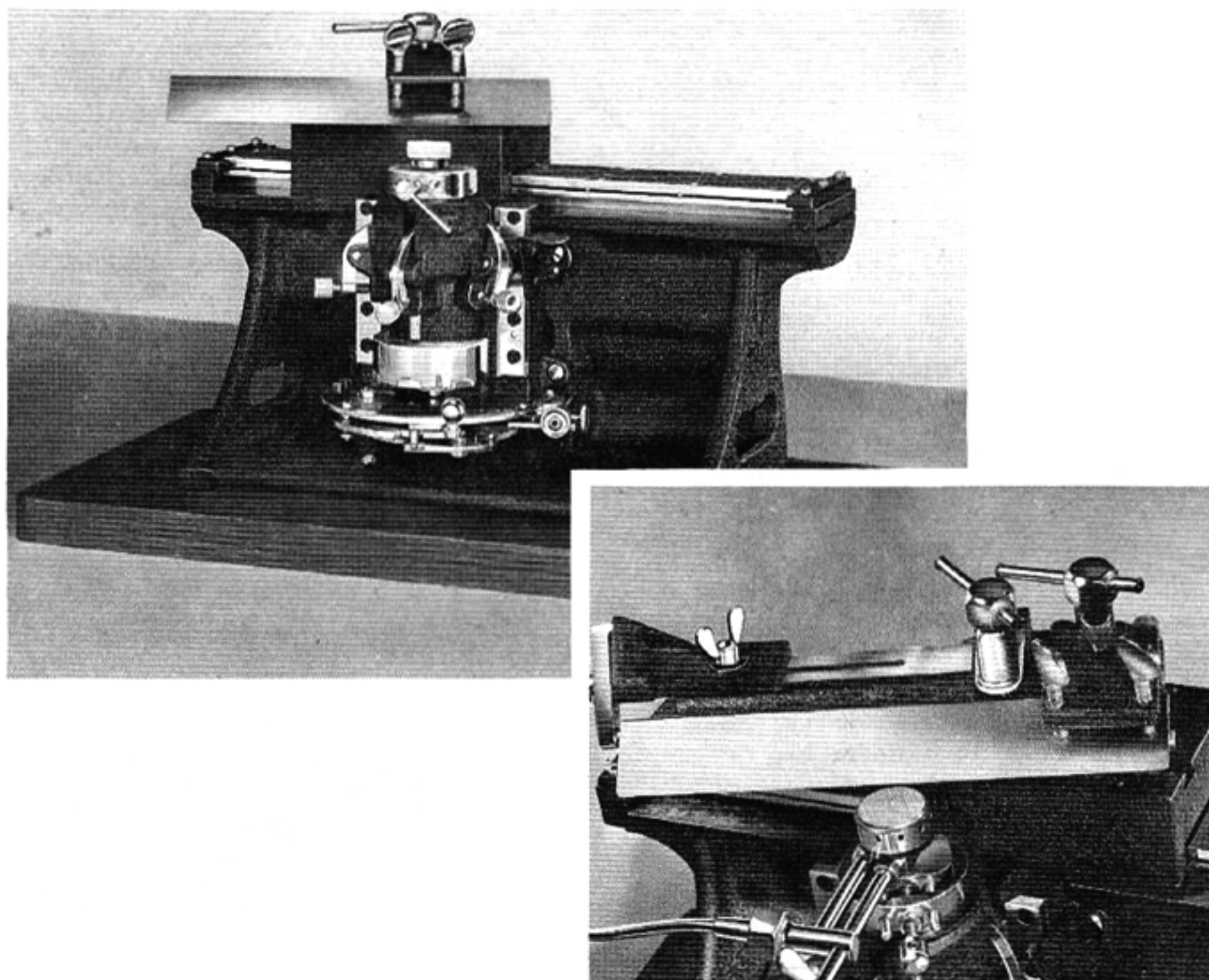
Fig. 17. AO 860 Sliding Microtome.
